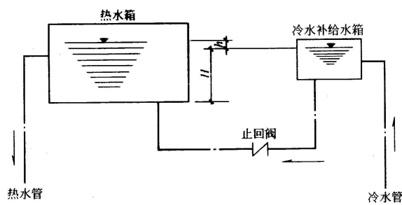
图8 热水箱与冷水补给水箱布置
