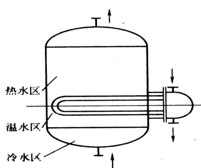
图 5 容积式加热器
