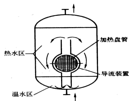
图 6 带导流装置的容积式加热器
